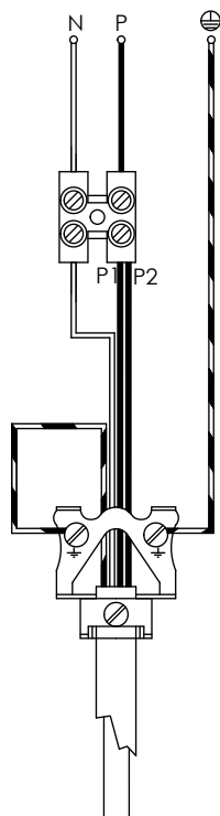
1 Stromkreis
