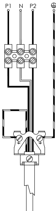
2 Stromkreise
