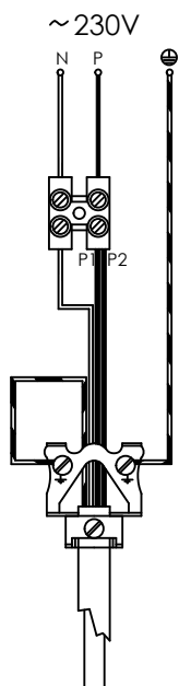
1 Stromkreis
