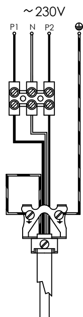
2 Stromkreise
